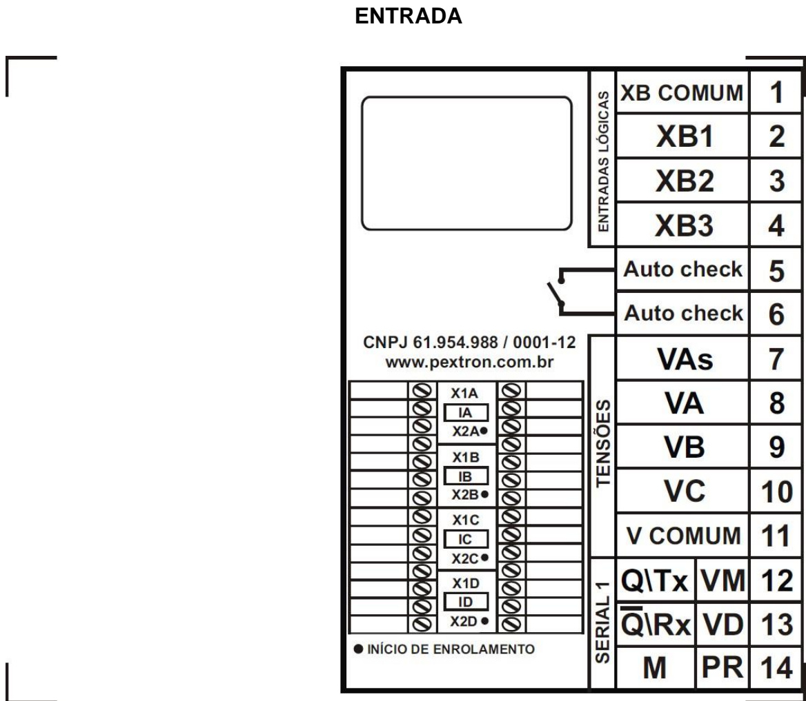
Figura 25.1: Bornes das entradas URP640x.
