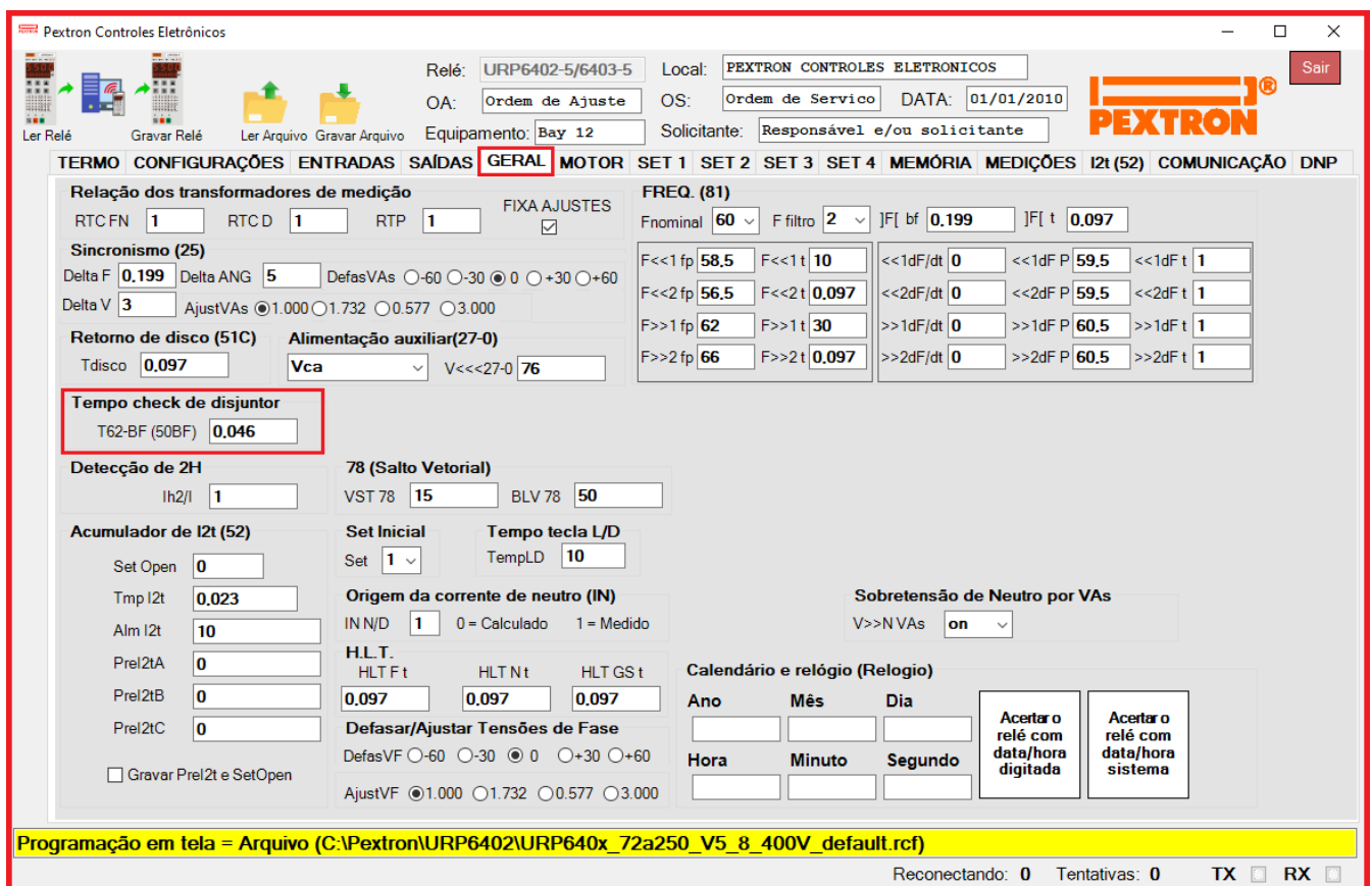
Figura 16.1: Pasta GERAL sinalizando a unidade de falha do disjuntor.
