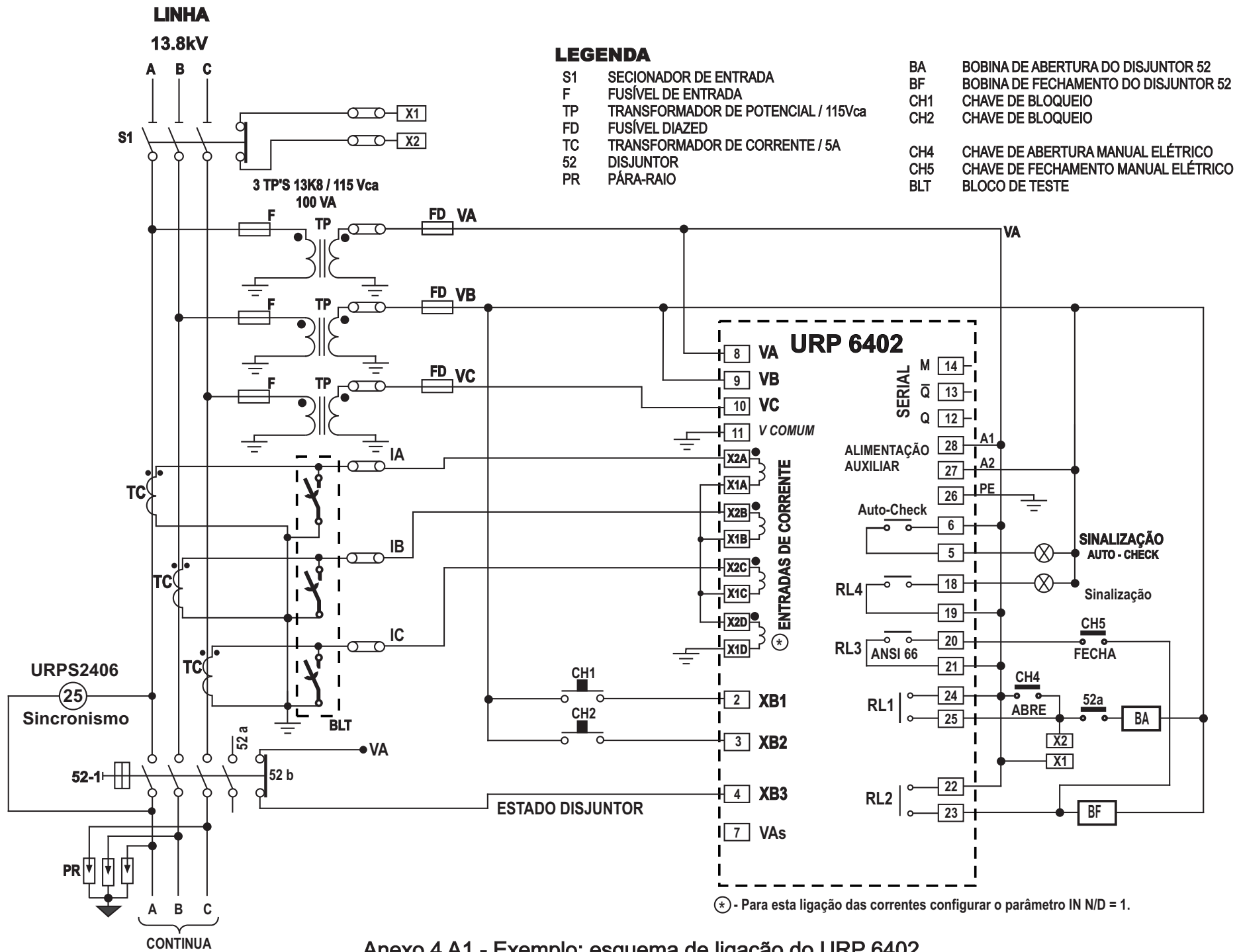
Anexo 4 A1 - Exemplo: esquema de ligação do URP 6402.
