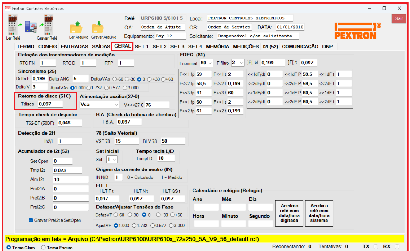
Figura 8.9: Pasta GERAL sinalizado com o parâmetro da unidade de sobrecorrente com controle de torque (51C).
