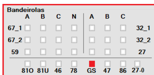
Figura 8.6: Pasta MEDIÇÕES sinalização do sensor de terra.
