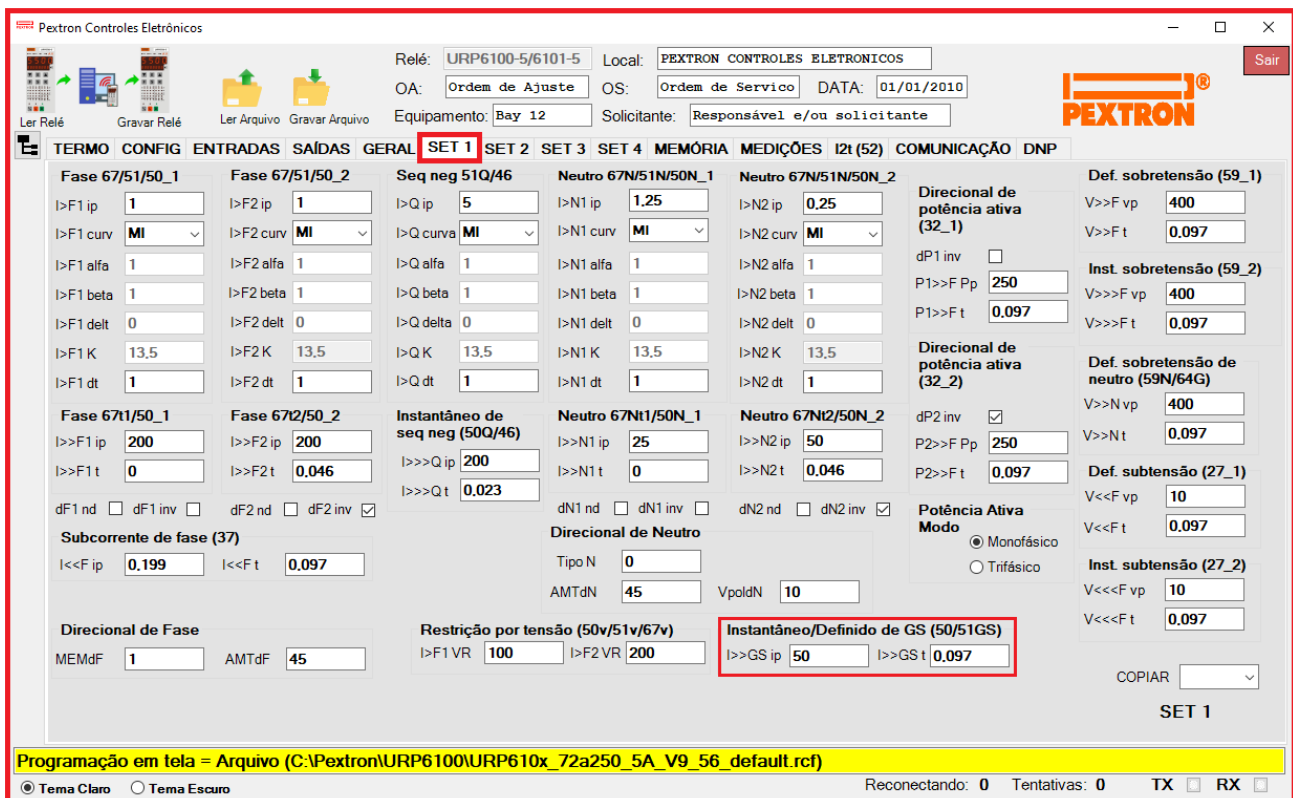
Figura 8.5: Pasta SET 1 sinalizando a unidade temporizada de tempo definido.
