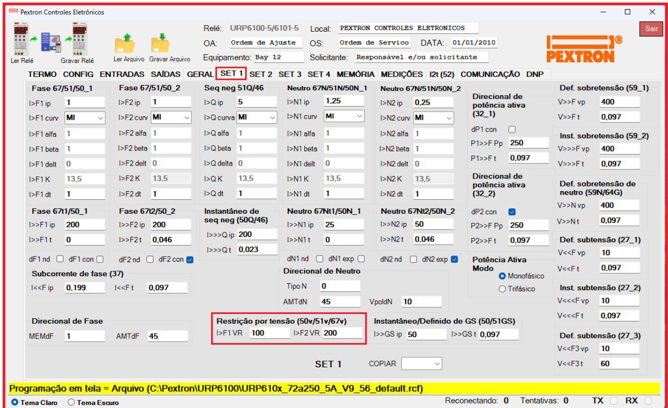
Figura 8.7: Pasta SET 1 sinalizando a unidade de sobrecorrente tempo dependente com restrição por tensão.
