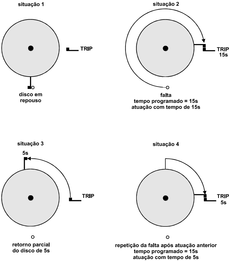
Figura 8.10: Simulação da atuação de relé eletromecânico.
