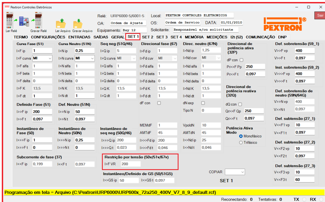
Figura 8.6: Pasta SET 1 sinalizando a unidade de restrição de sobrecorrente de fase por tensão.
