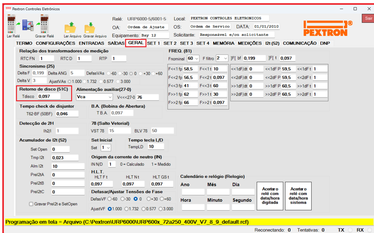
Figura 8.8: Pasta GERAL sinalizando a unidade de sobrecorrente com controle de torque (51C).
