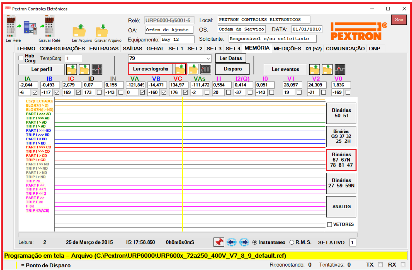
Figura 21.7: Registro de Oscilografia para exibir as binárias 67 / 67N / 78 / 81 / 47.
