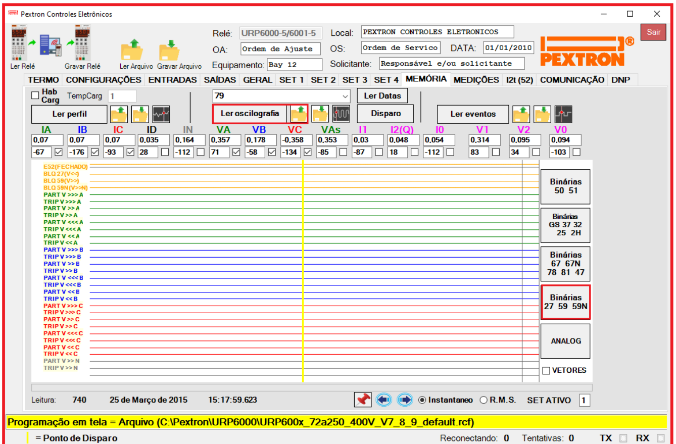
Figura 21.8: Registro de Oscilografia para exibir as binárias 27 / 59 / 59N selecionadas.
