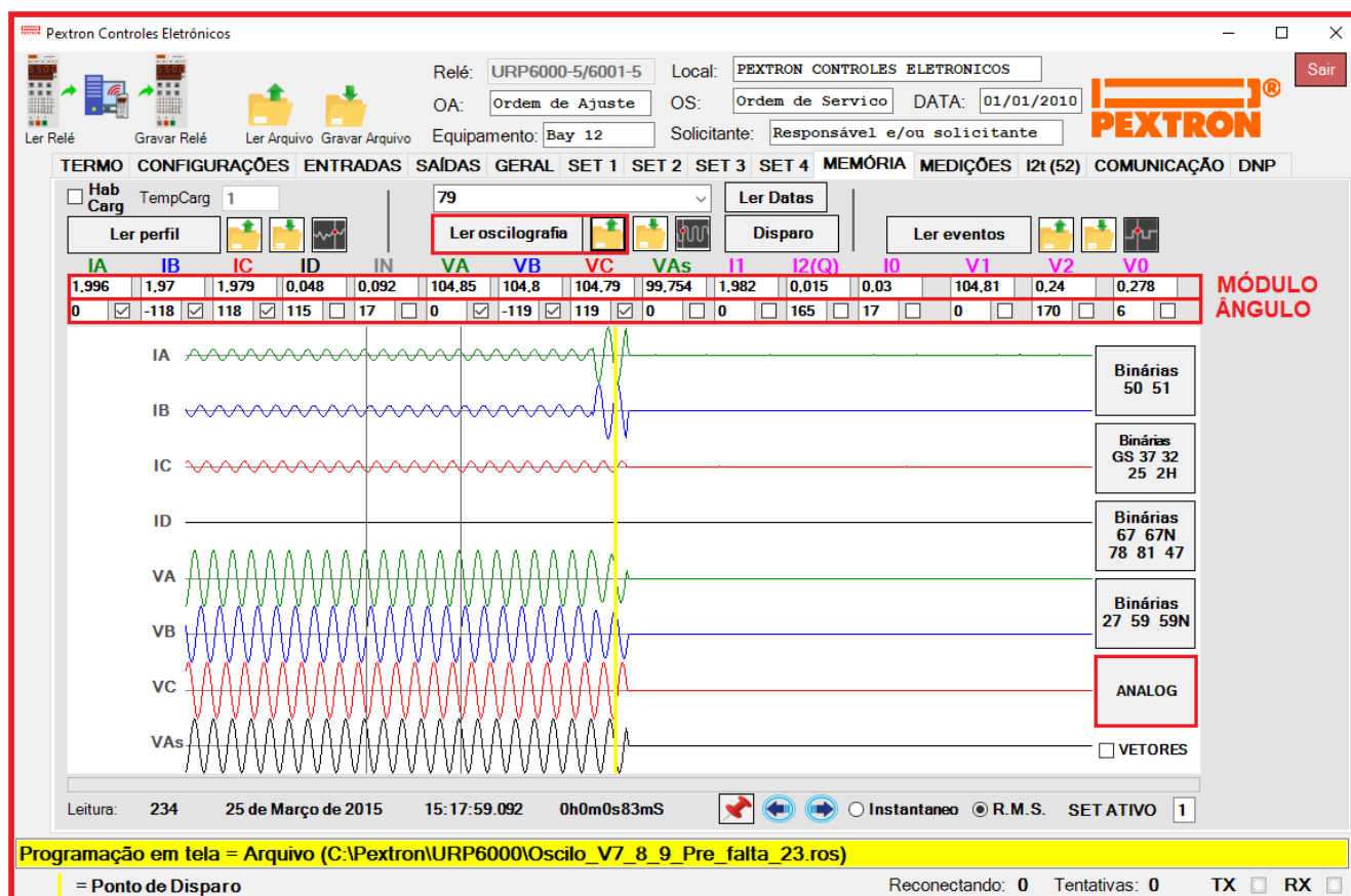
Figura 21.2: Pasta MEMÓRIA com leitura de registro de oscilografia.
