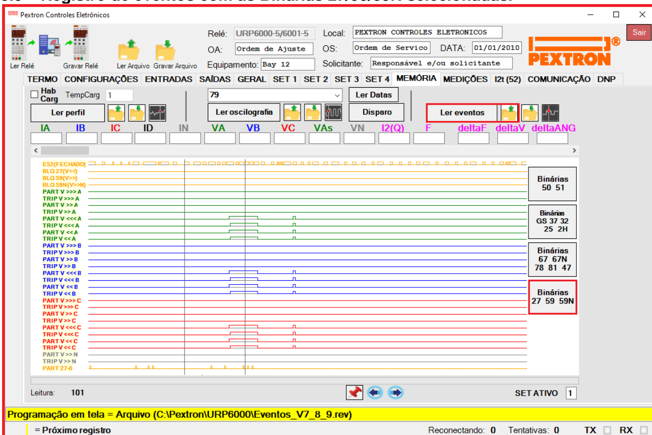
Figura 21.15: Registro de eventos nas funções binárias 27 / 59 / 59N.
