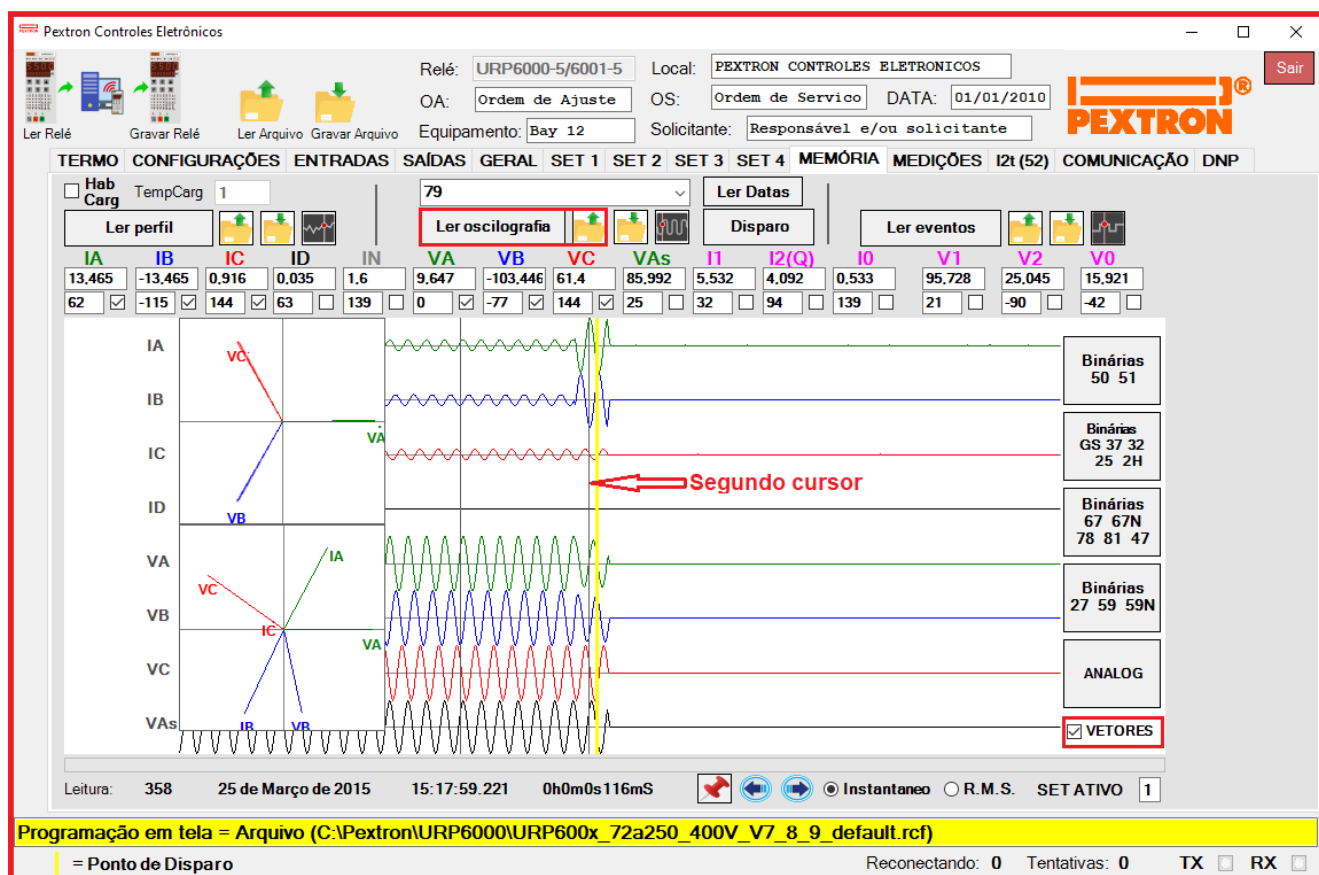
Figura 21.10: Exibição do segundo quadro dos Fasores.
