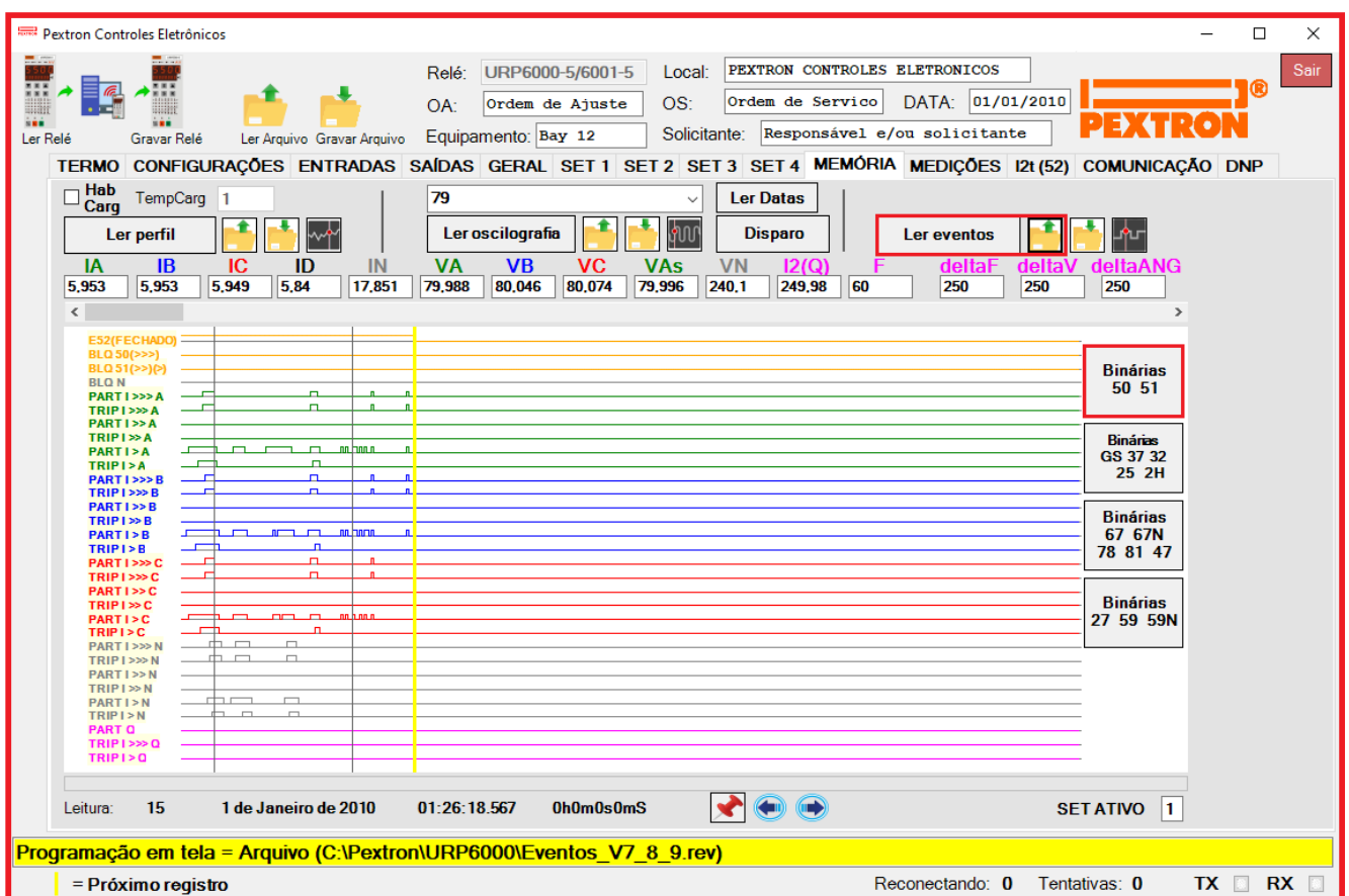
Figura 21.11: Pasta MEMÓRIA o com leitura de registro de eventos (Binárias 50 / 51) .
