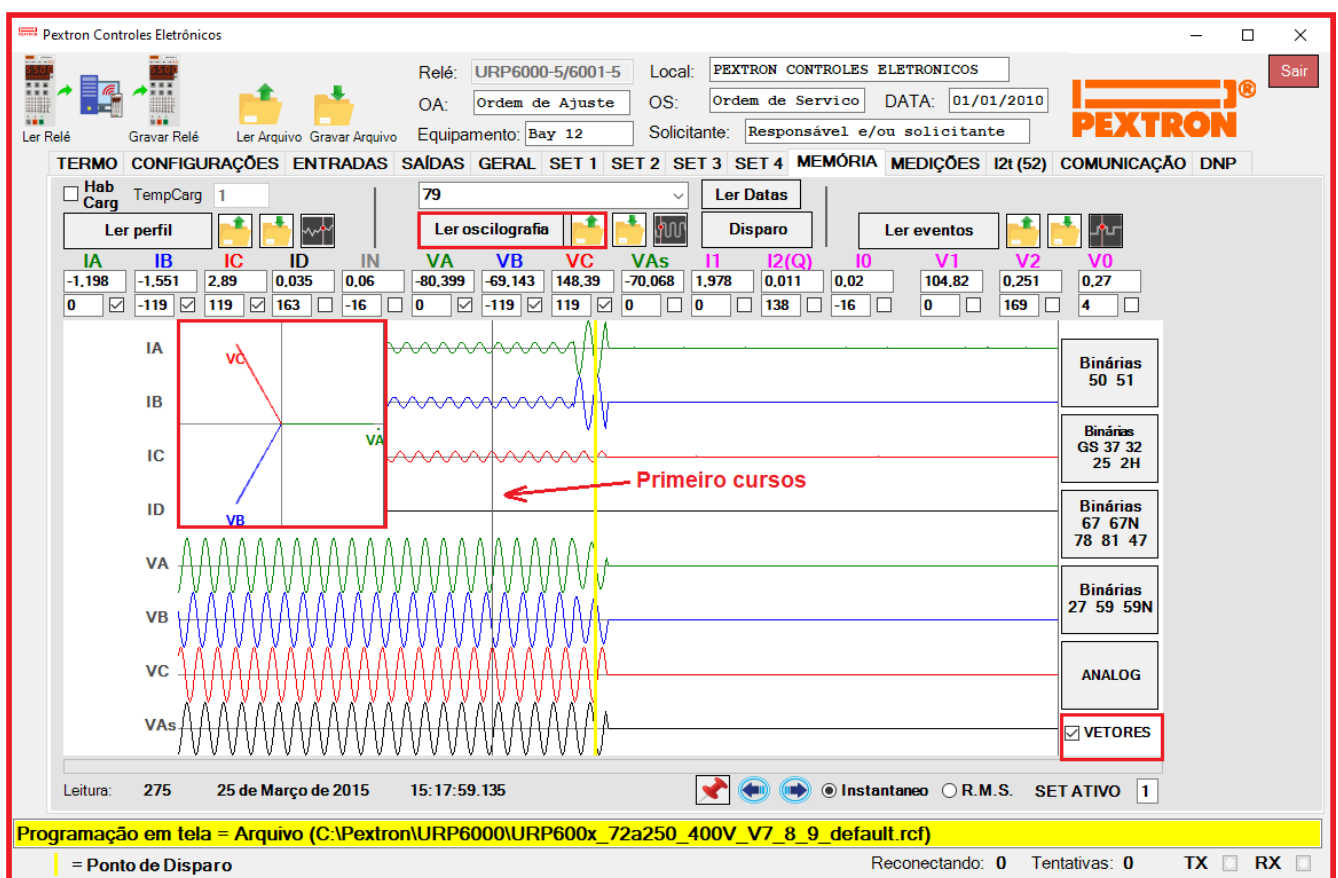
Figura 21.9: Exibição do quadro dos Fasores para o primeiro cursor
