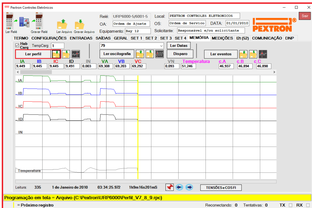
Figura 21.1: Pasta MEMÓRIA com leitura de registro de perfil de carga.
