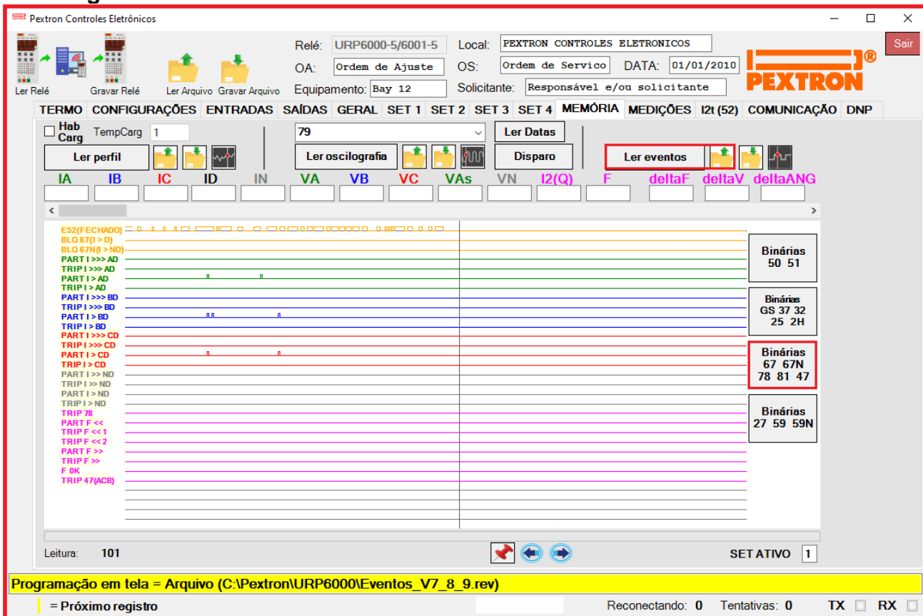
Figura 21.14: Registro de Eventos com as funções Binárias 67 / 67N/ 78 / 81 / 47 selecionadas.
