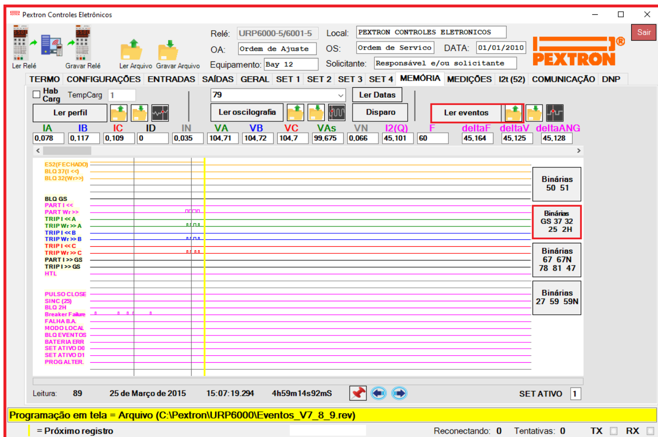
Figura 21.13: Registro de eventos nas funções binárias GS / 37 / 32 / 25 / 2H.
