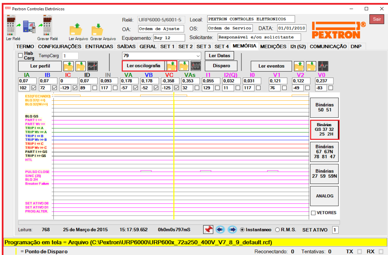
Figura 21.6: Registro de Oscilografia para exibir as binárias GS/ 37 / 32 / 25 / 2h.
