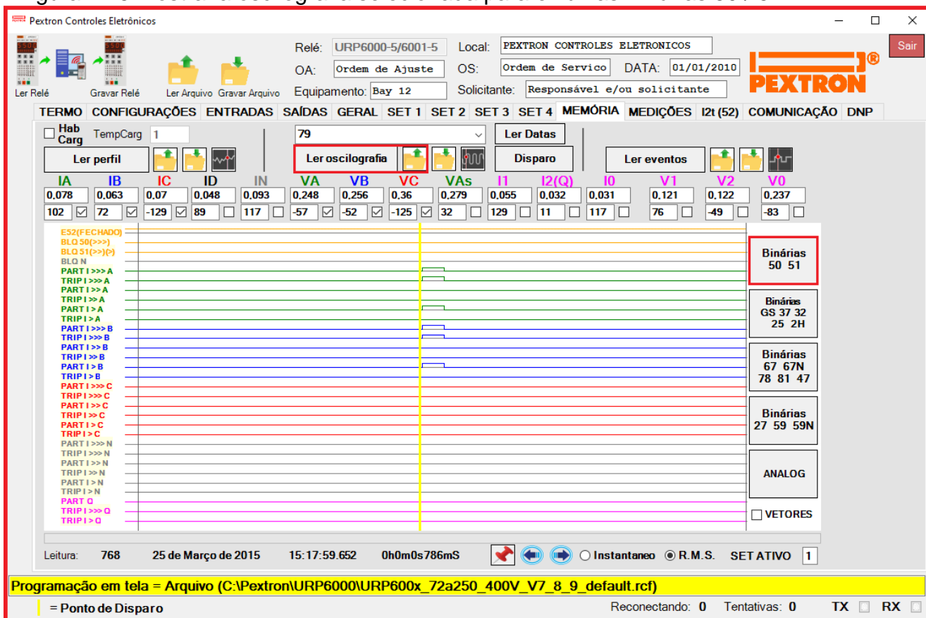
Figura 21.5: Registro de Oscilografia para exibir as funções binárias 50/51.
