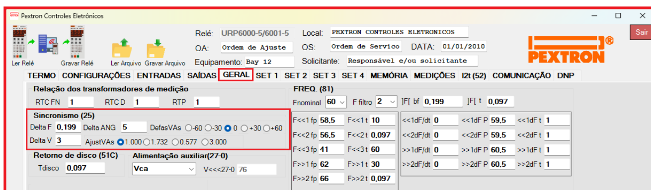
Figura 13.1: Pasta GERAL sinalizado com os parâmetros da unidade de sincronismo.
