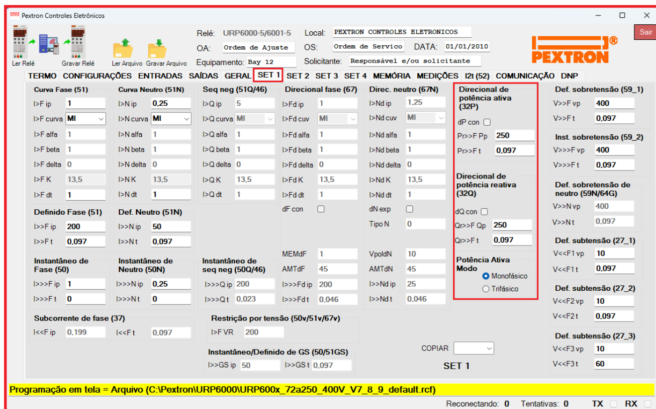
Figura 10.9: Pasta SET 1 do programa aplicativo sinalizando a unidade direcional de potência.
