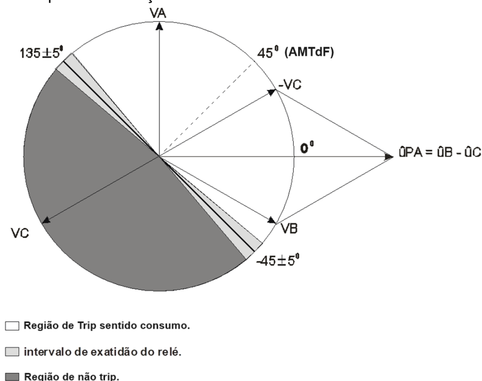
Figura 10.3: Diagrama fasorial da unidade direcional (67) em modo consumo com ângulo de máximo torque 45^\circ para a fase A com reversão de plano.
