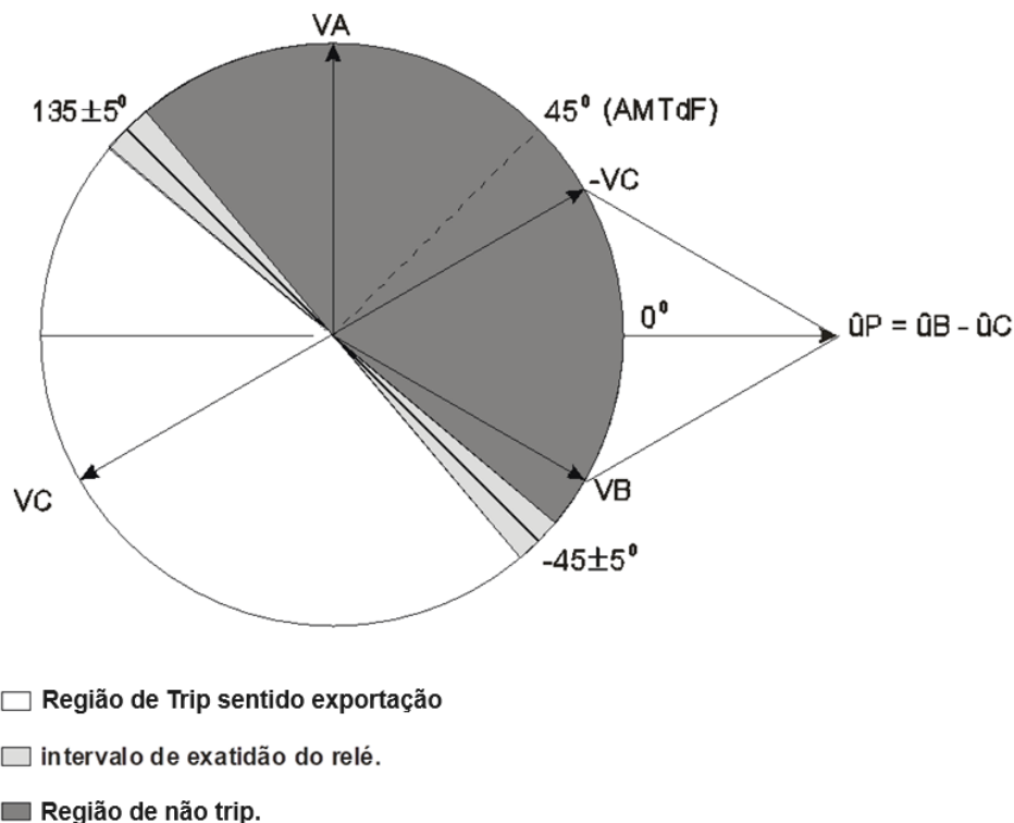
Figura 10.2: Diagrama fasorial da unidade direcional (67) em modo exportação com ângulo de máximo torque 45^\circ para a fase A.
