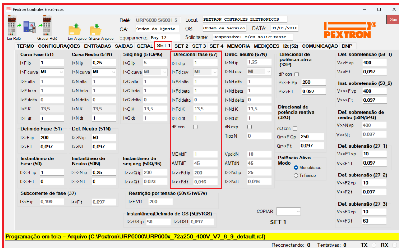
Figura 10.1: Pasta SET 1 sinalizando a unidade de sobrecorrente direcional de fase.
